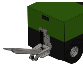
Artikel H0128-D35 Klapphaken Ø35
