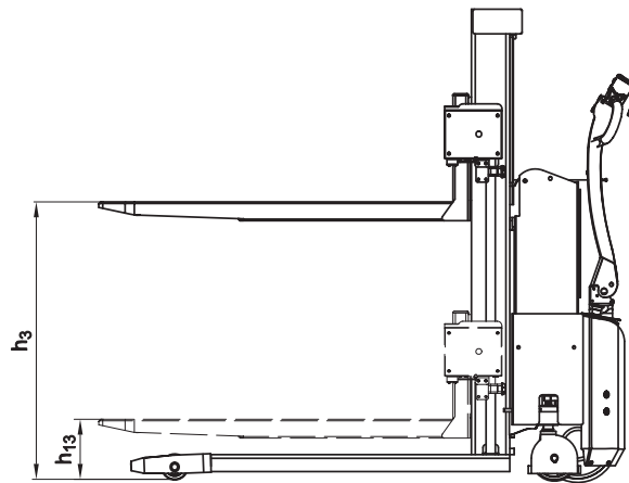
Positionskontrolle hier am Elektro-Logiflex angebaut. Lässt sich auch an Elektro-Scherenhubwagen und Logiflex-Stapler anbauen.
