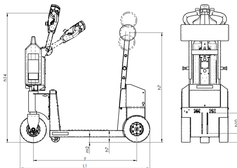
Abbildung 19. Produktabmessungen (Seiten- und Rückansicht)
