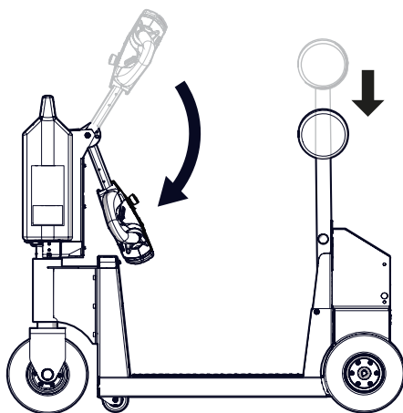
Abbildung 16. Transport des Produkts
