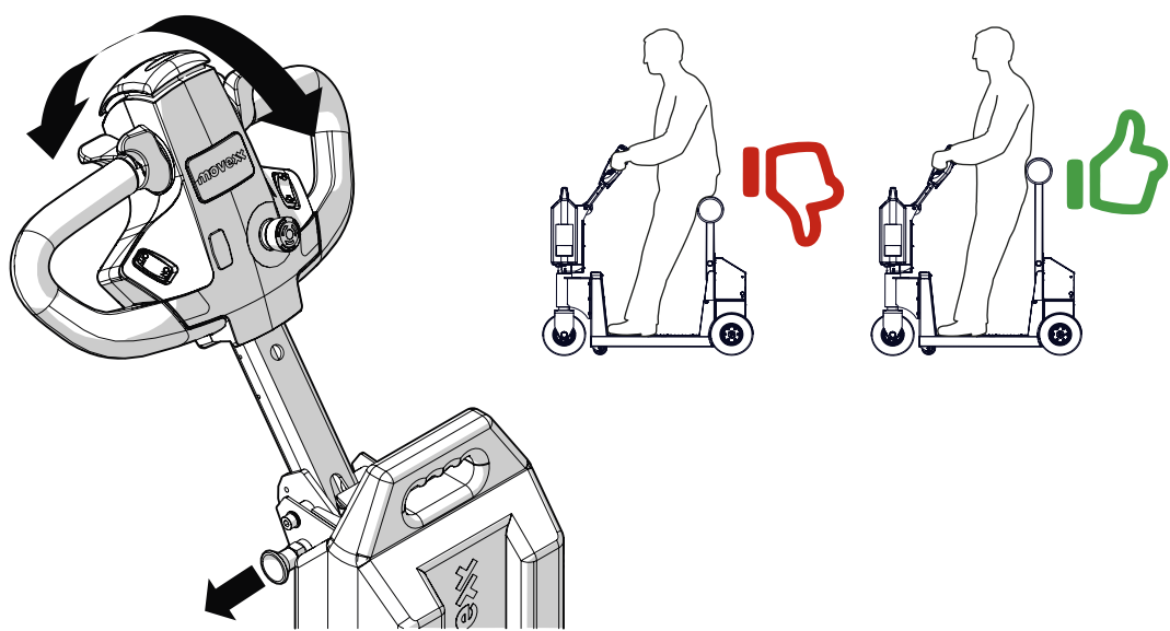
Abbildung 7. Höhe des Deichselkopfes
