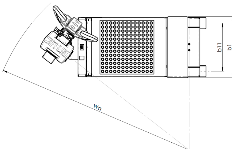
Abbildung 18. Produktabmessungen (Ansicht von oben)
