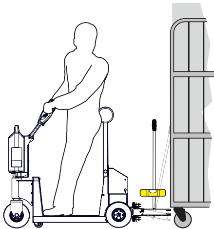
Abbildung 10. Anschließen der Last
