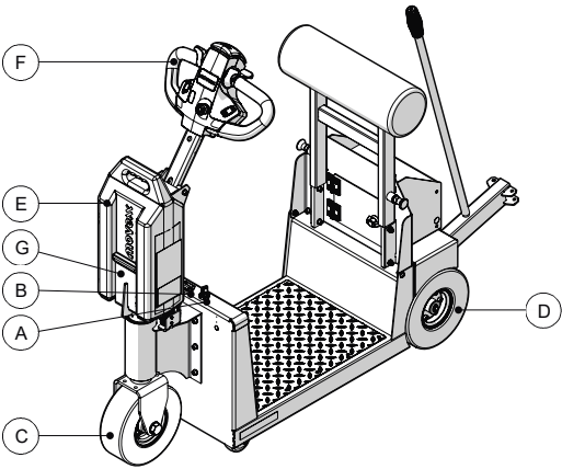
Abbildung 1. Produktübersicht
