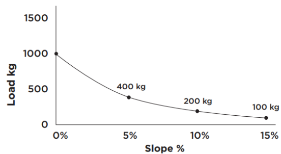
Abbildung 17. Maschinenkapazität
