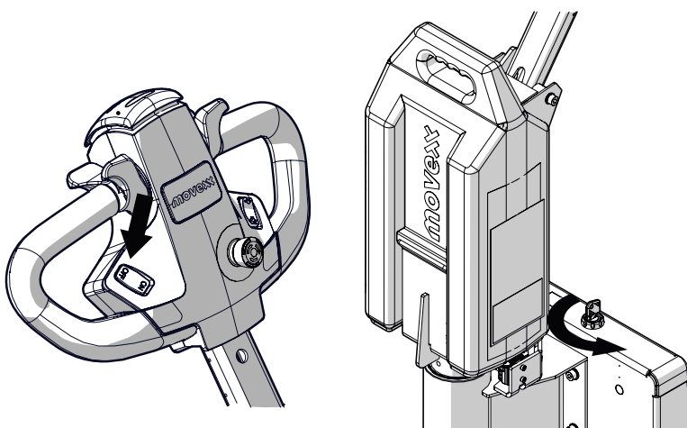
Abbildung 5. Ausschalten des Produkts
