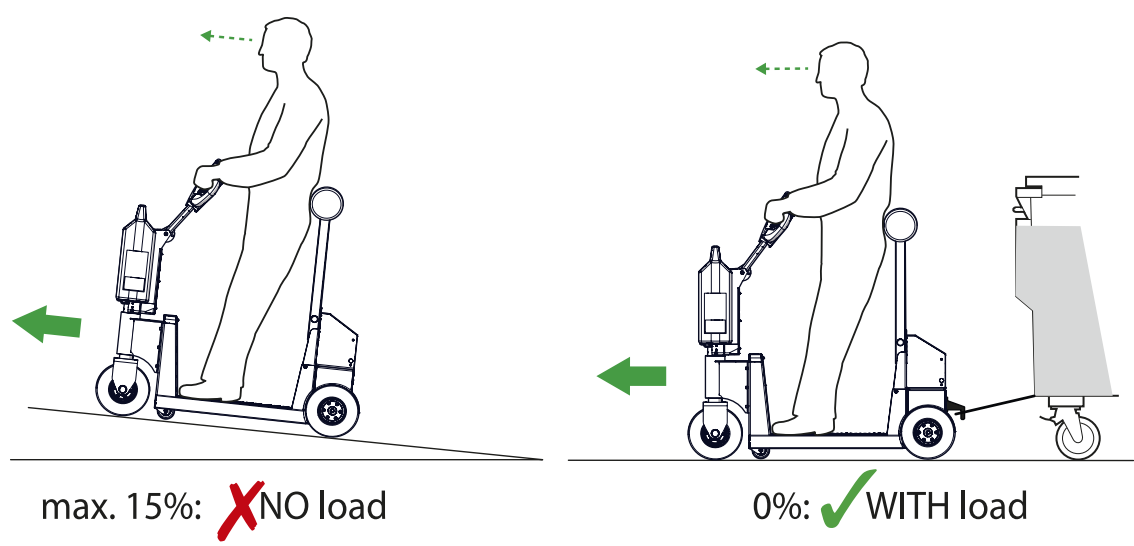
Abbildung 6. Fahren an Abhängen. Geringere Belastung an Hängen. Siehe Tabelle Maschinenkapazität.
