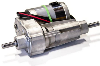
Artikel M1032 Motor 300W 100 U/min, ohne Feststellbremse
