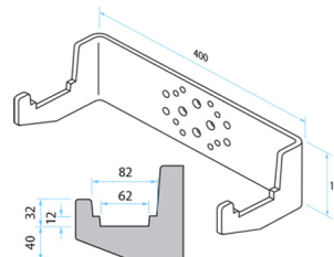
Artikel 335868 MD Standard 60-80 inkl. Kontraplt.
