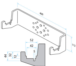
Artikel 335863 MD Standard 5-40-50 inkl. Kontraplt.
